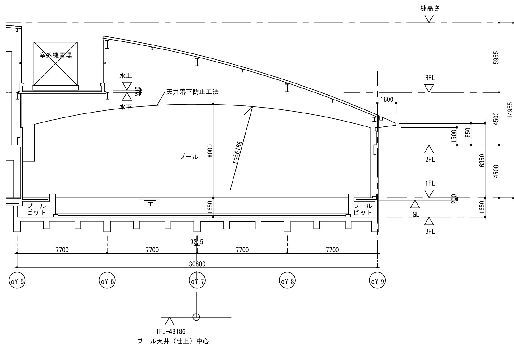
E-E断面図
