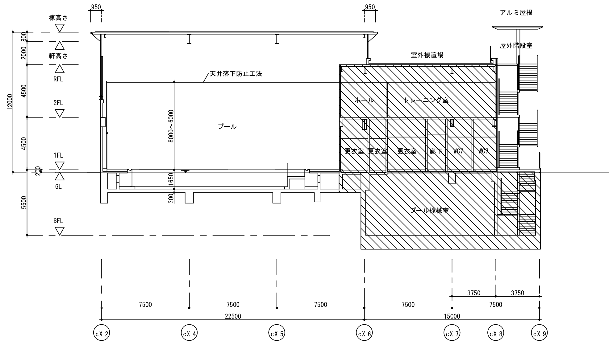
D-D断面図
